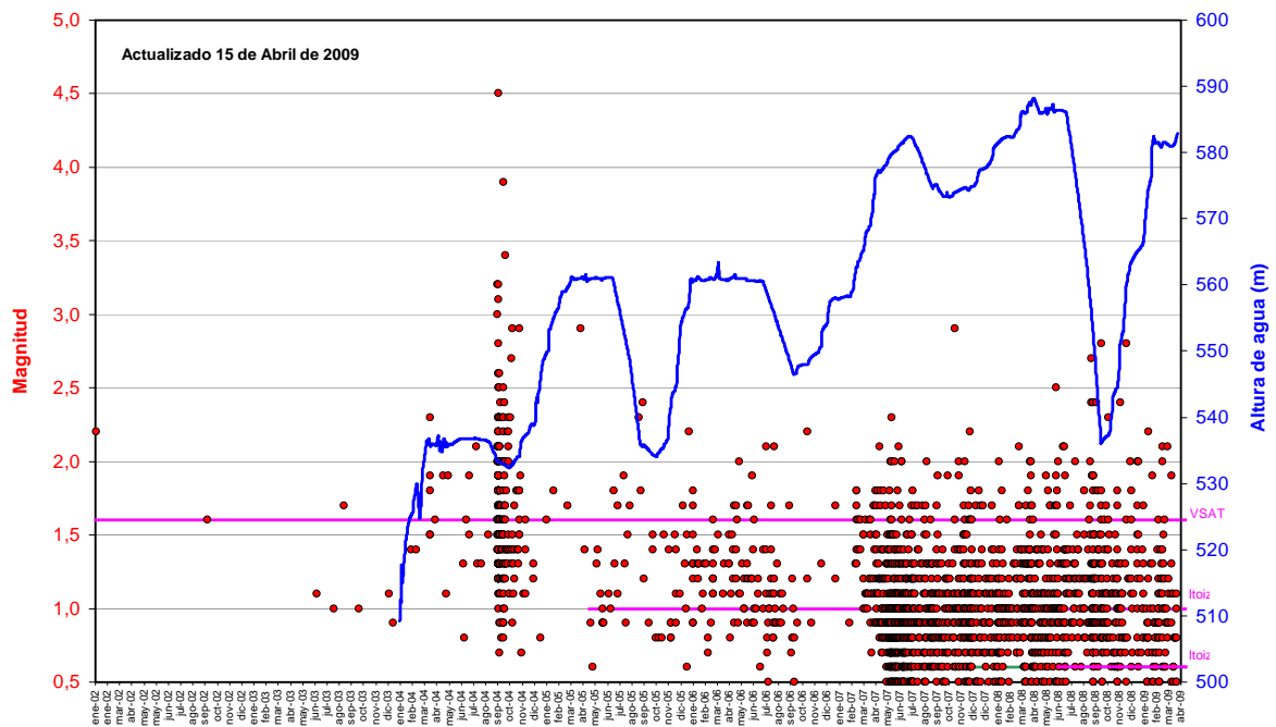
Figura 5.- Distribución temporal de los terremotos localizados en el periodo desde el 1 de enero de 2002 al 15 de abril de 2009 en la zona limitada por los paralelos 42,7N-43,0N y los meridianos 1,6W-1,1W, junto con la curva de llenado.
