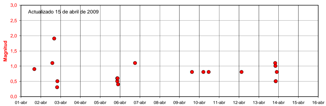
Figura 4.- Distribución temporal de los terremotos localizados en el periodo del 01 al 15 de abril de 2009 en la zona limitada por los paralelos 42,7N-43,0N y los meridianos 1,6W-1,1W.
