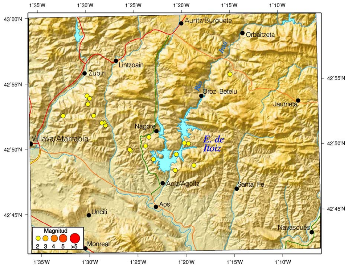
Figura 3.- Terremotos localizados en el periodo del 01 al 15 de abril de 2009 en la zona limitada por los paralelos 42,7N-43,0N y los meridianos 1,6W-1,1W.
